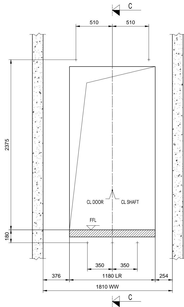
Otvori za vrata u vaznom oknu Pogled iz vaznog okna Stanice: -1, 0, 1, 2 - Strana A
