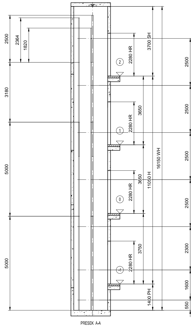
PRESEK A-A
