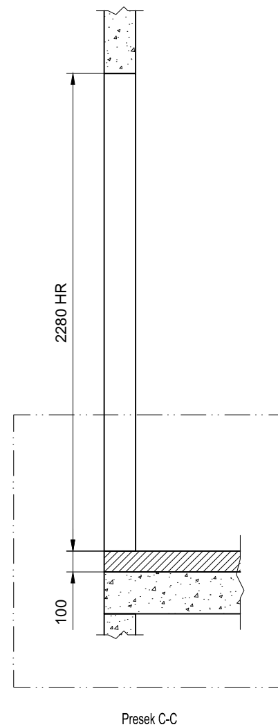
Presek C-C
