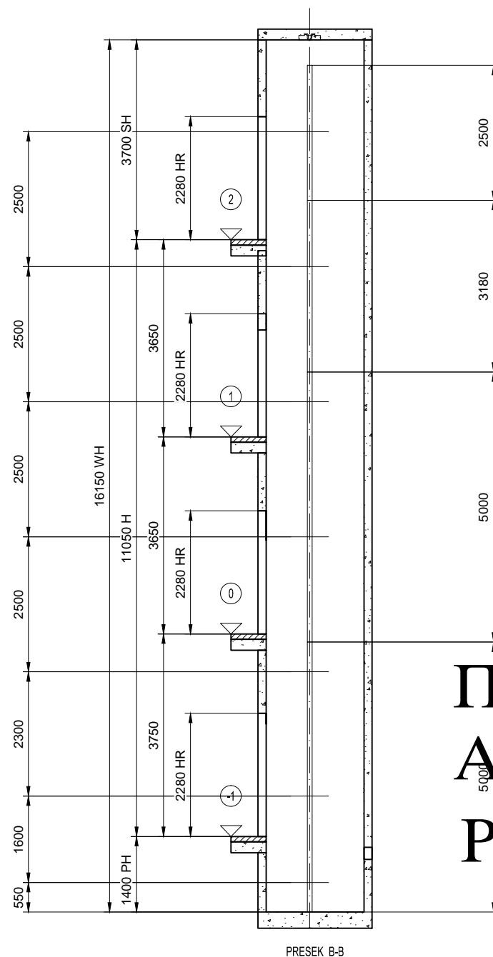
PRESEK B-B
