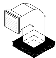
Primer izvođenja zaštite otvora za ventilaciju / informativno
