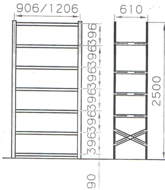
Presek poličnih regala na pozicijama 3 i 4
