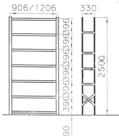
Presek poličnih regala na pozicijama 1i2
