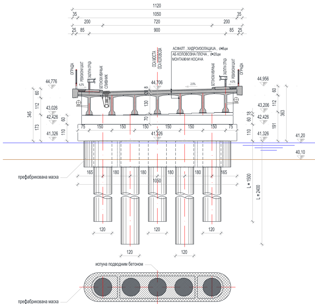
Прилог 5 – Попречни пресеци моста - новопроектовано стање
