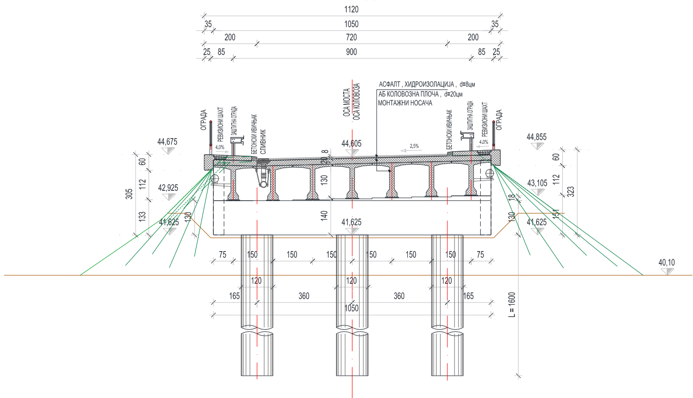
Прилог 6 – Попречни пресеци моста - новопроектирано стање
