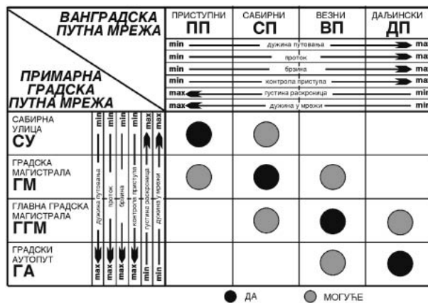
Слика 5-03: Општи принцип повезивања ванградске и градске путне мреже сагласно одговарајућим функционалним класификацијама.
