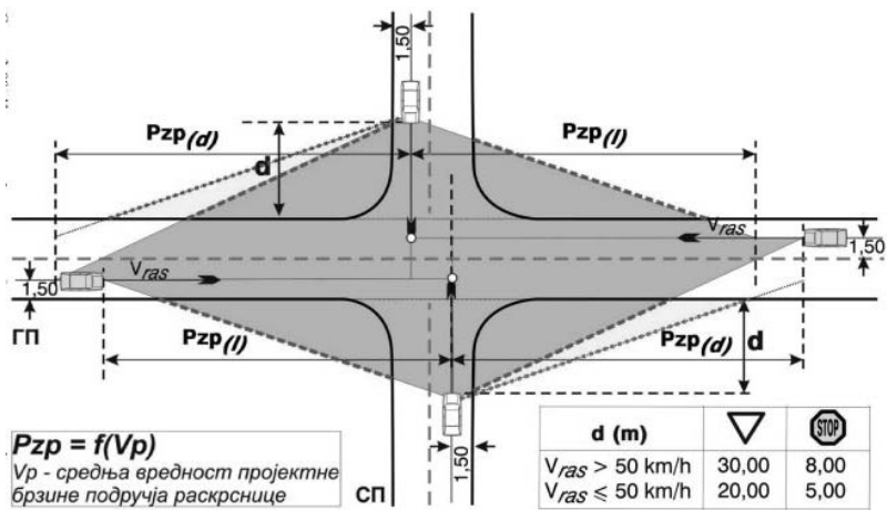
Слика 3-09: Конструкција зона прегледности на четворокракој површинској раскрсници.
