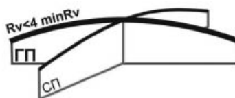
Слика 2-08: Услови за избор локације површинске раскрснице у ситуационом плану и подужном профилу.
