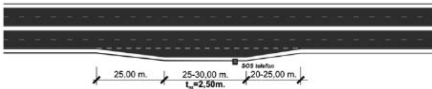
Слика 5-05: Стандардни облик нише за зауостављање возила.
