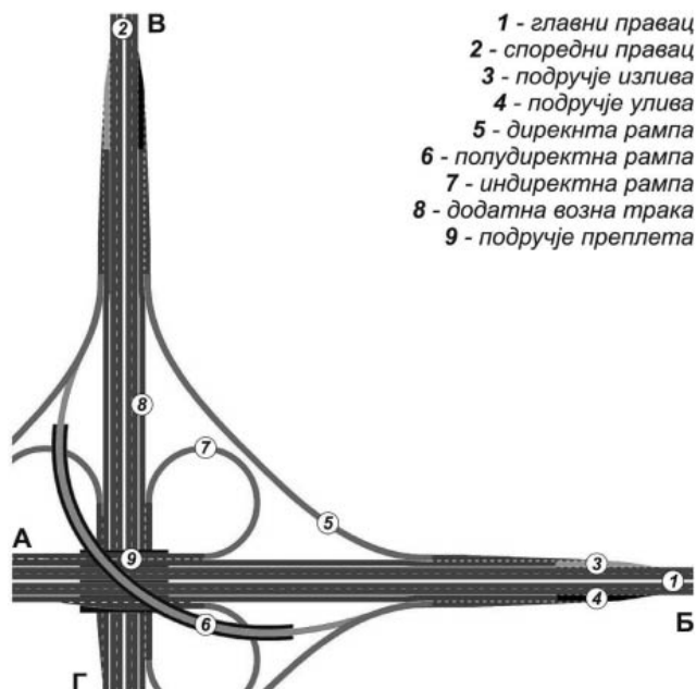
Слика 2-01: Основни елементи денivelисане раскрснице.
