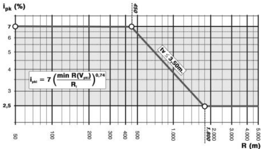
Слика 8-01: Номограм за одређивање величине попречног нагиба коловоза у кривинама (двотрачни путеви и вишетрачни путеви).
