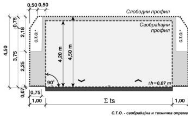
Слика 5-12: Слободни и саобраћајни профил двотрачног / вишетрачног пута.
