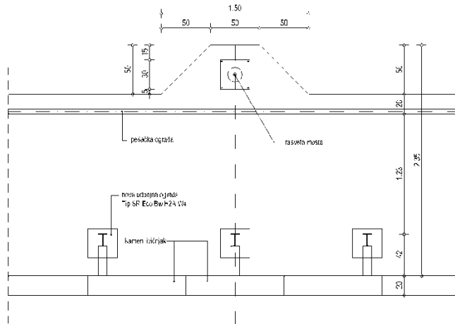
DETALJ 'C' VIČNI VENAC SA PROŠIRENJEJ ZA RASVETU R. 120
