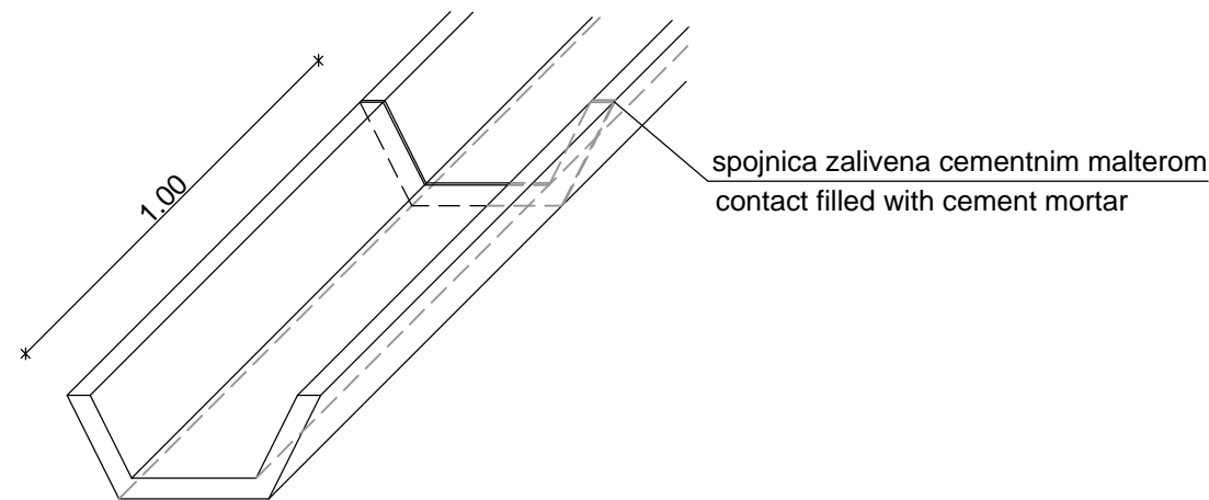
AKSONOMETRIJA AXONOMETRY
