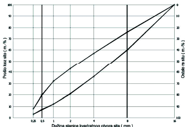
Slika 2.3.5: Granične krive granulometrijskog sastava za smese kamenih zrna za mešavine cementnog betona CB 32
